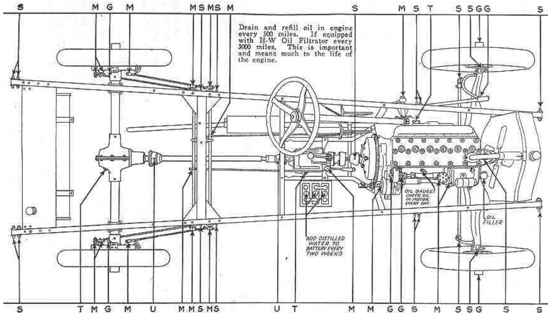
Fig. 85—Lubrication Chart
